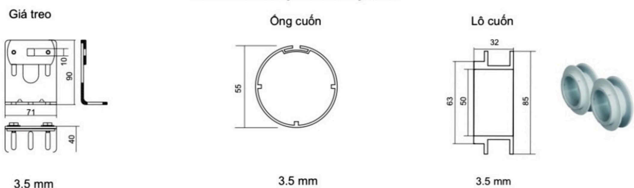
Bản mô tả mặt cắt sản phẩm
