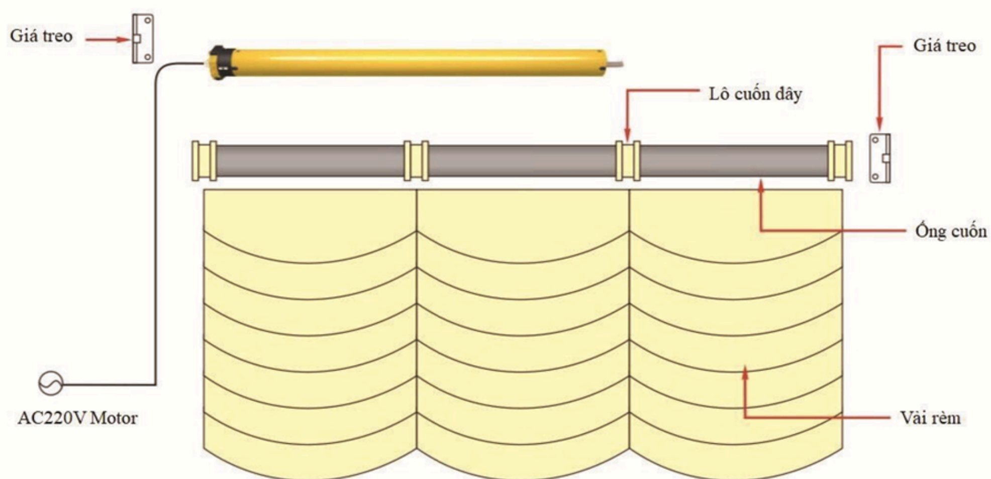
Bản mô tả mặt cắt sản phẩm
