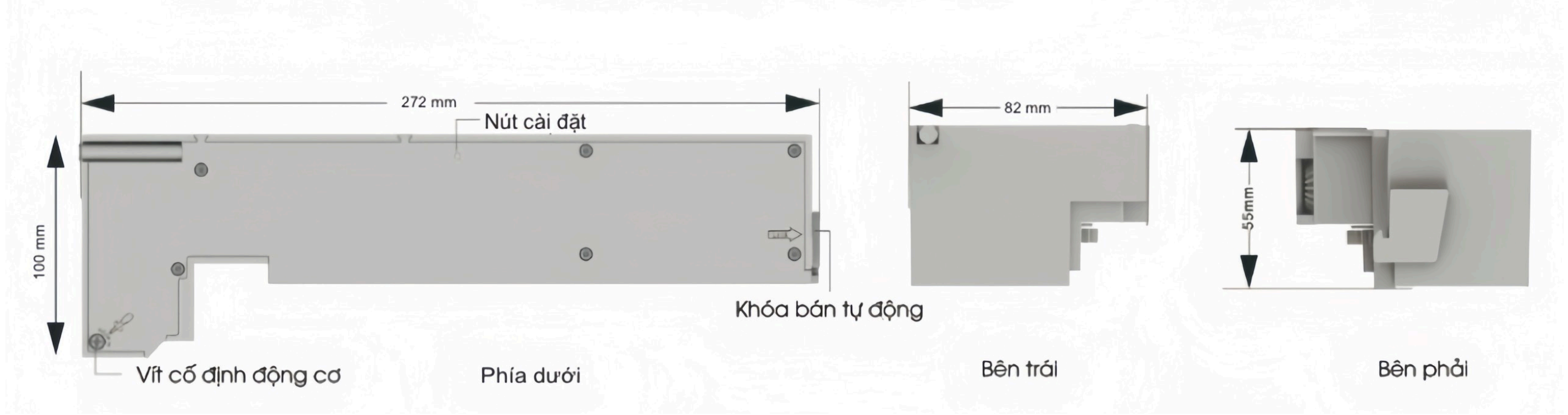
Bản mô tả mặt cắt sản phẩm
