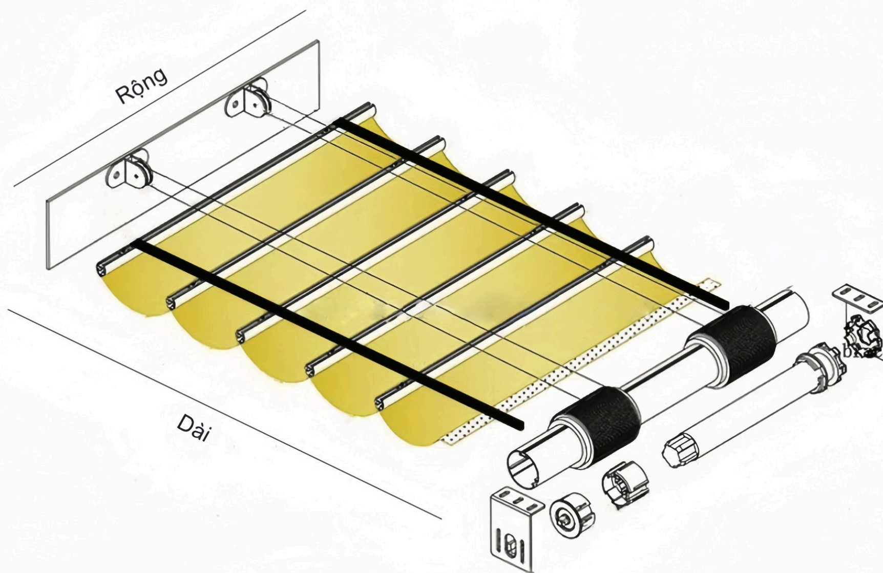
Bản mô tả mặt cắt sản phẩm
