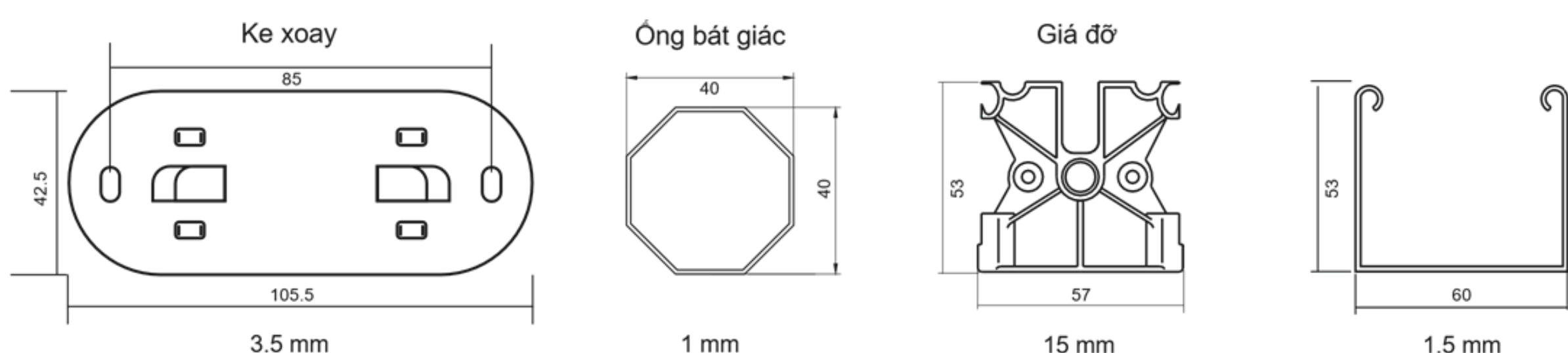
Bản mô tả mặt cắt sản phẩm
